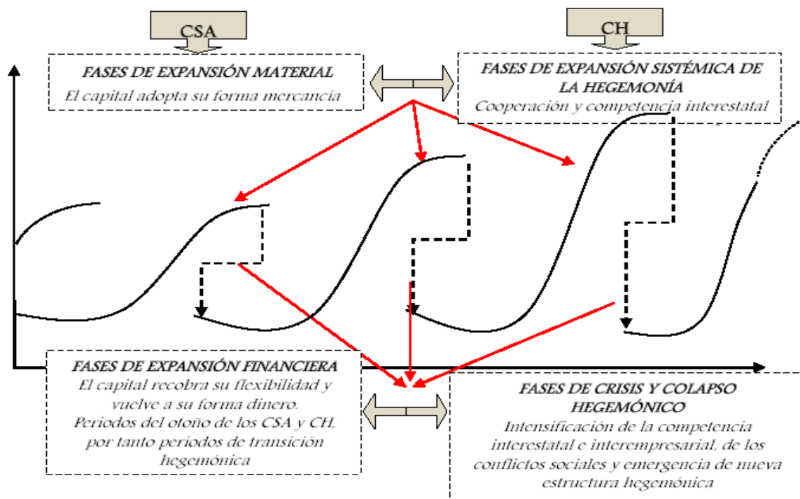
Gráfico: csa y ch en el planteamiento arrighiano
