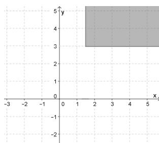
Figura 11.7: Fórmula:
