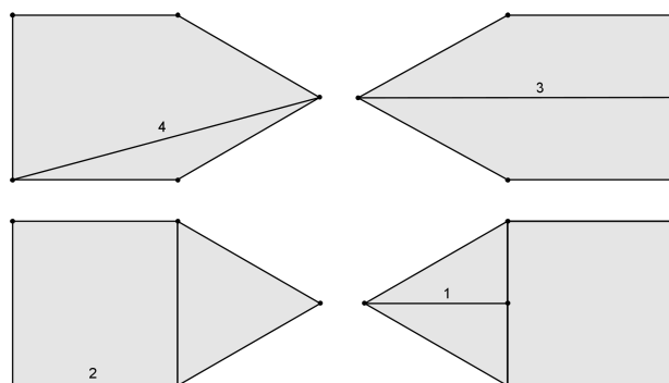
Figura 11.3: Pentágonos equiláteros
