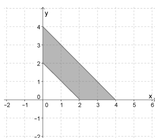
Figura 11.9: Fórmula:
