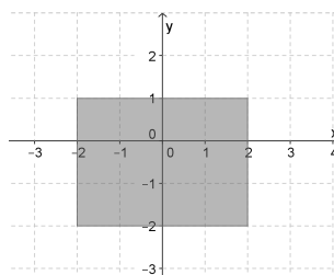
Figura 11.14: Fórmula:
